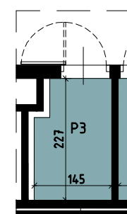
Komórka lokatorska P3 Komórka lokatorska 3.02
