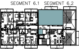
Piętro 6
